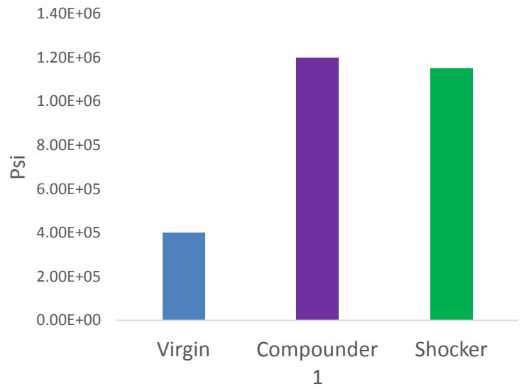
Tensile Modulus (Psi)
